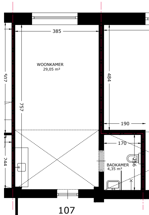
BEGANE GROND
